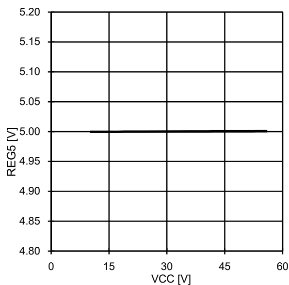
Fig.26 REG5-VCC
