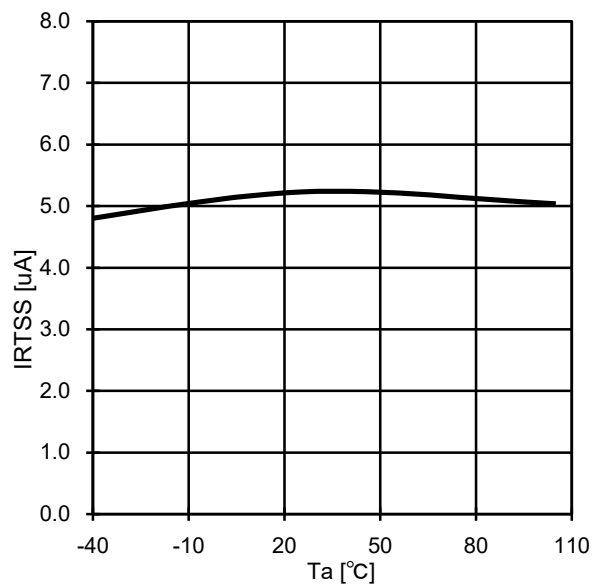
Fig.3 IRTSS-Ta (VRTSS=0V)
