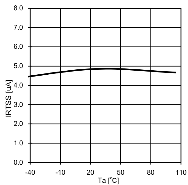
Fig.4 IRTSS-Ta (VRTSS=1V)
