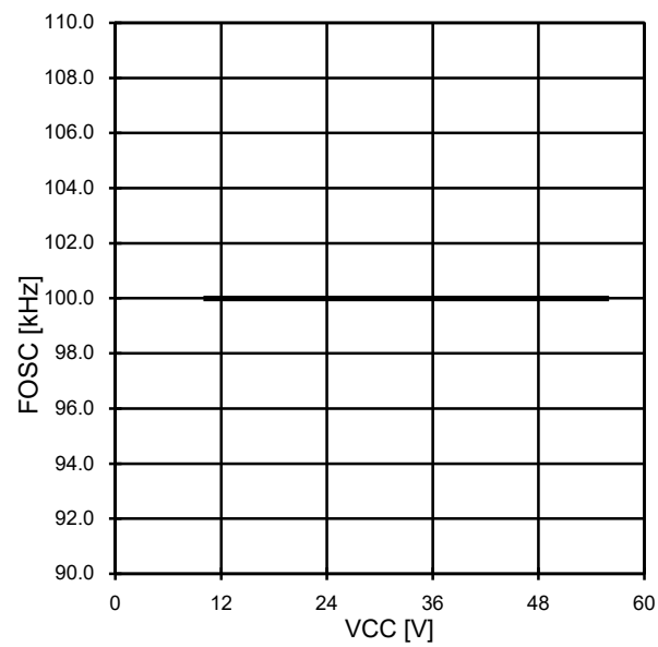
Fig.2 FOSC-VCC
