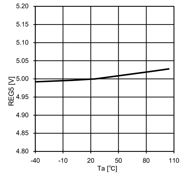
Fig.25 REG5-Ta
