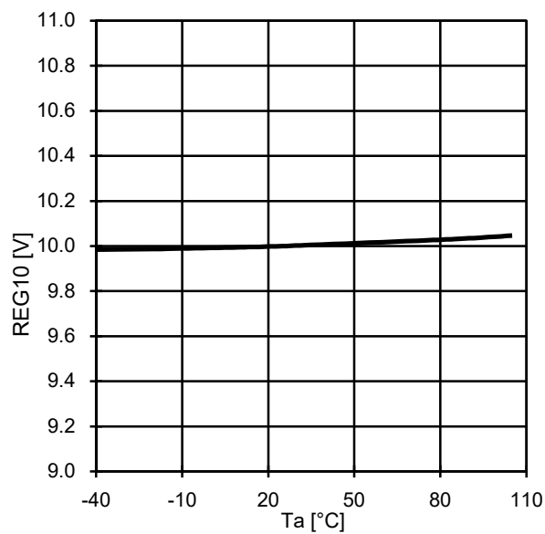
Fig.23 REG10-Ta
